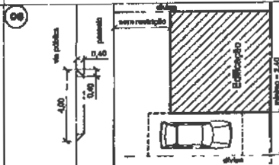
Imóvel com testada inferior a 8,00m, existentes na data da publicação da Lei Complementar nº 418/04.
