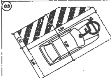
Dimensão mínima da vaga de auto para deficientes (inclinação)
