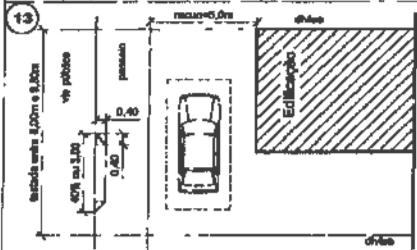
Situação não permitida para imóvel com testada entre 8,00m e 9,50m.
