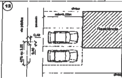
Situação permitida em residência unifamiliar.
