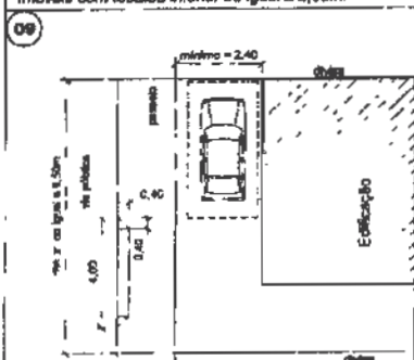
Estacionamento permitido para imóvel com testada maior ou igual a 9,50m
