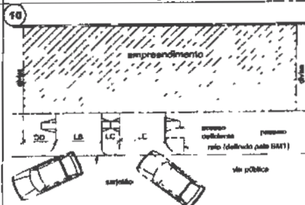
O rebatimento do passeio para acesso ao empreendimento quando permitido, deverá ser previamente aprovado pela S.M. de Transportes, e qual definirá: distância da divisa (D.O.), largura da entrada (L.E.), largura do centro (L.C.) e largura da saída (L.S.).
