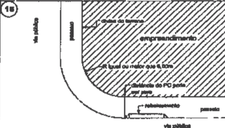
Rebatismo em esquina (raio maior ou igual a 6,00m)
