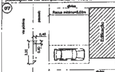
Imóvel com testada inferior ou igual a 8,00m.
