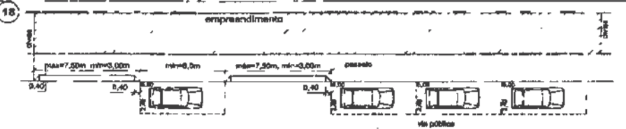
Imóvel com testada maior que 8,00m, a soma dos rebatimentos deverá ser igual ou inferior a 40% da testada.
